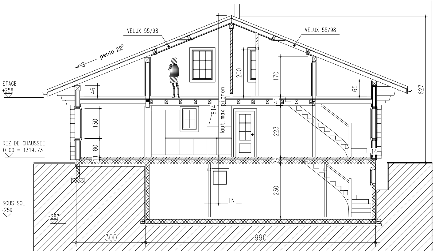
Coupe A-A
