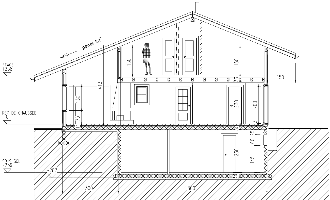
Coupe A-A
