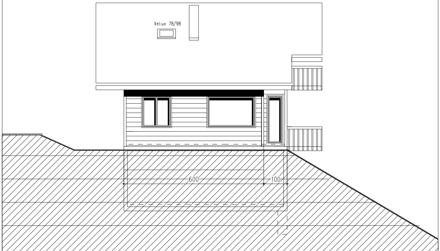
Facade Ouest
