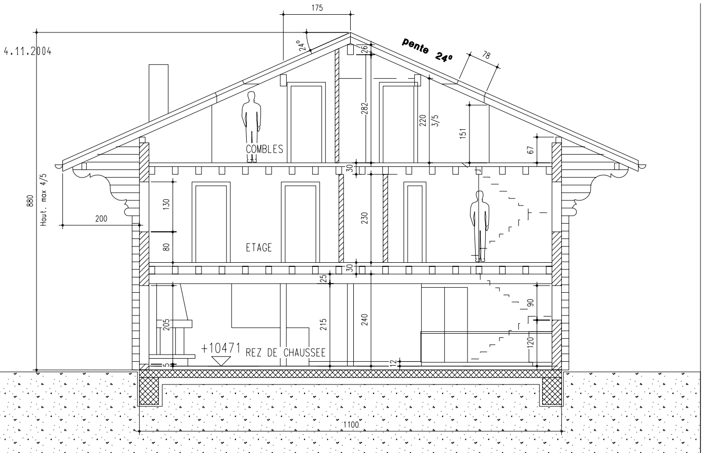
COUPE A-A
