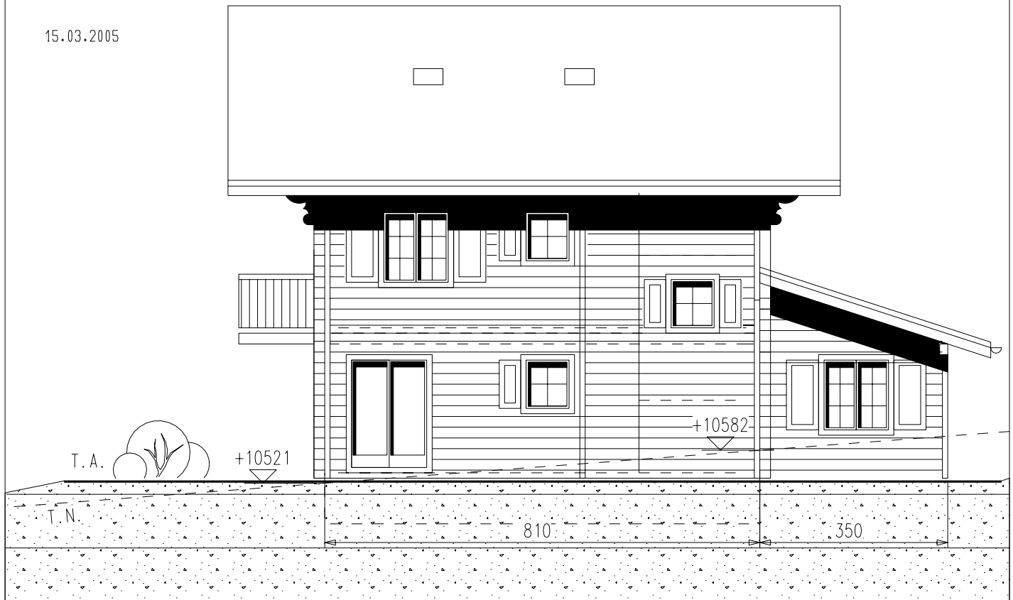
Facade EST
