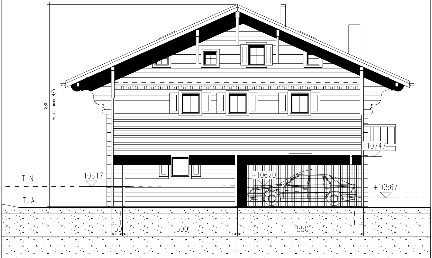
Facade NORD
