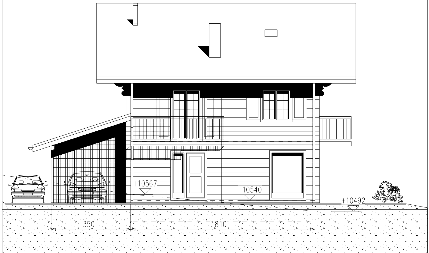
Facade OUEST
