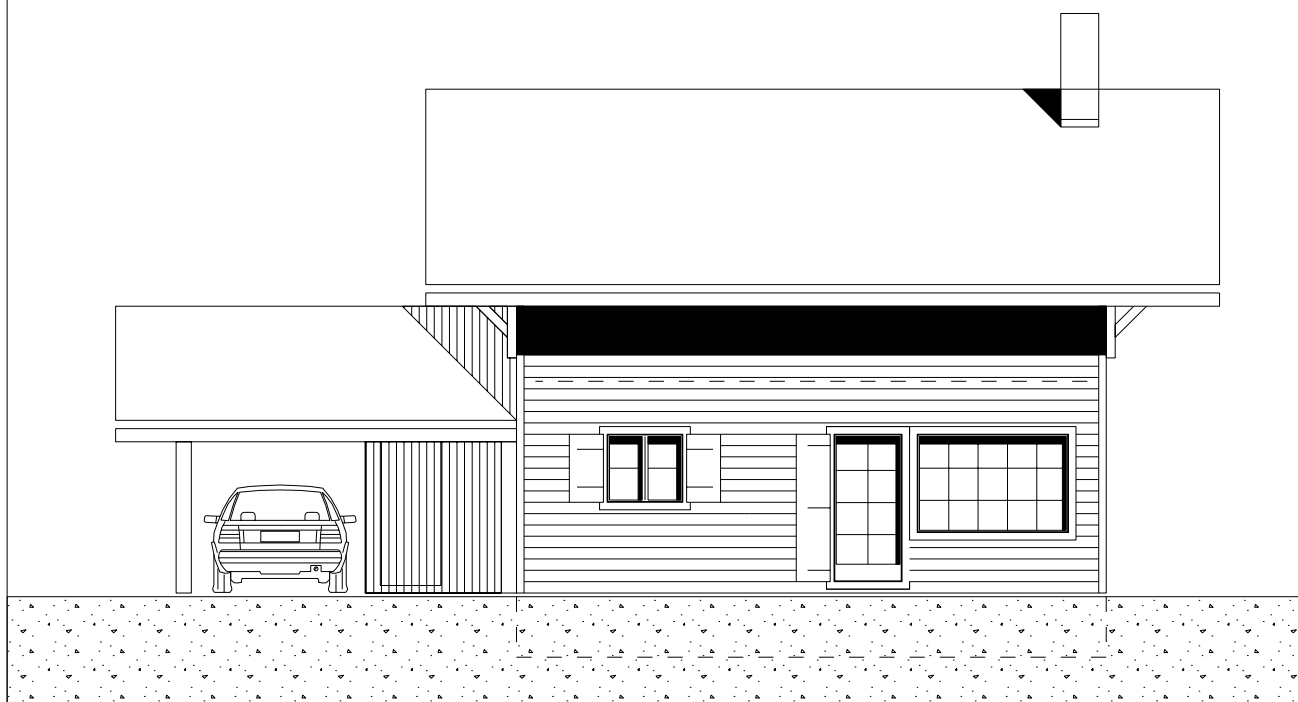
Facade Ouest
