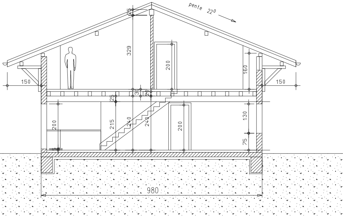
Coupe A-A
