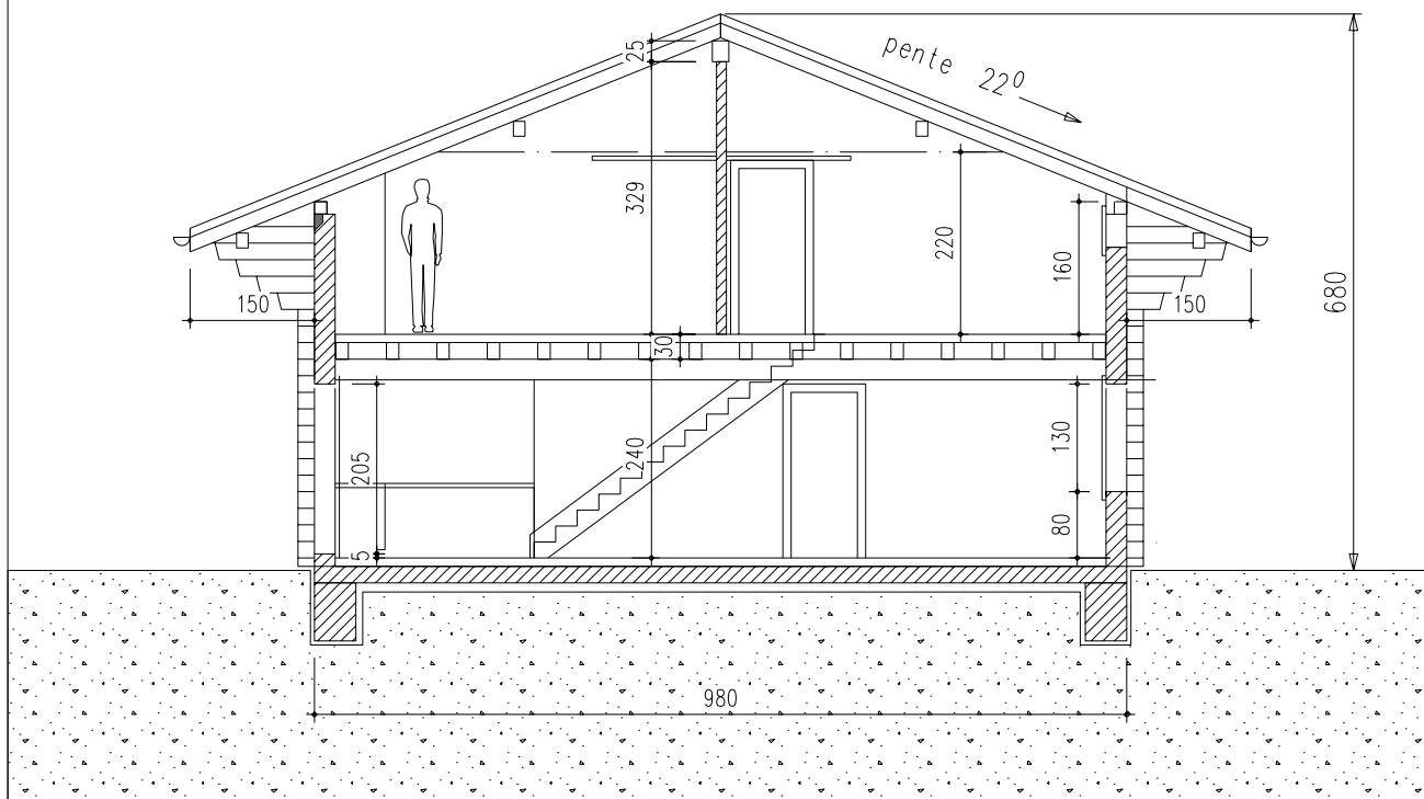
Coupe A-A
