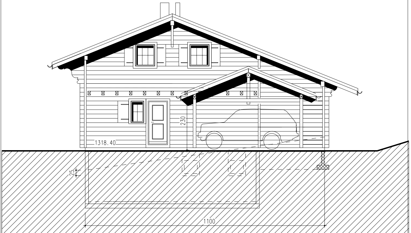
Facade Nord
