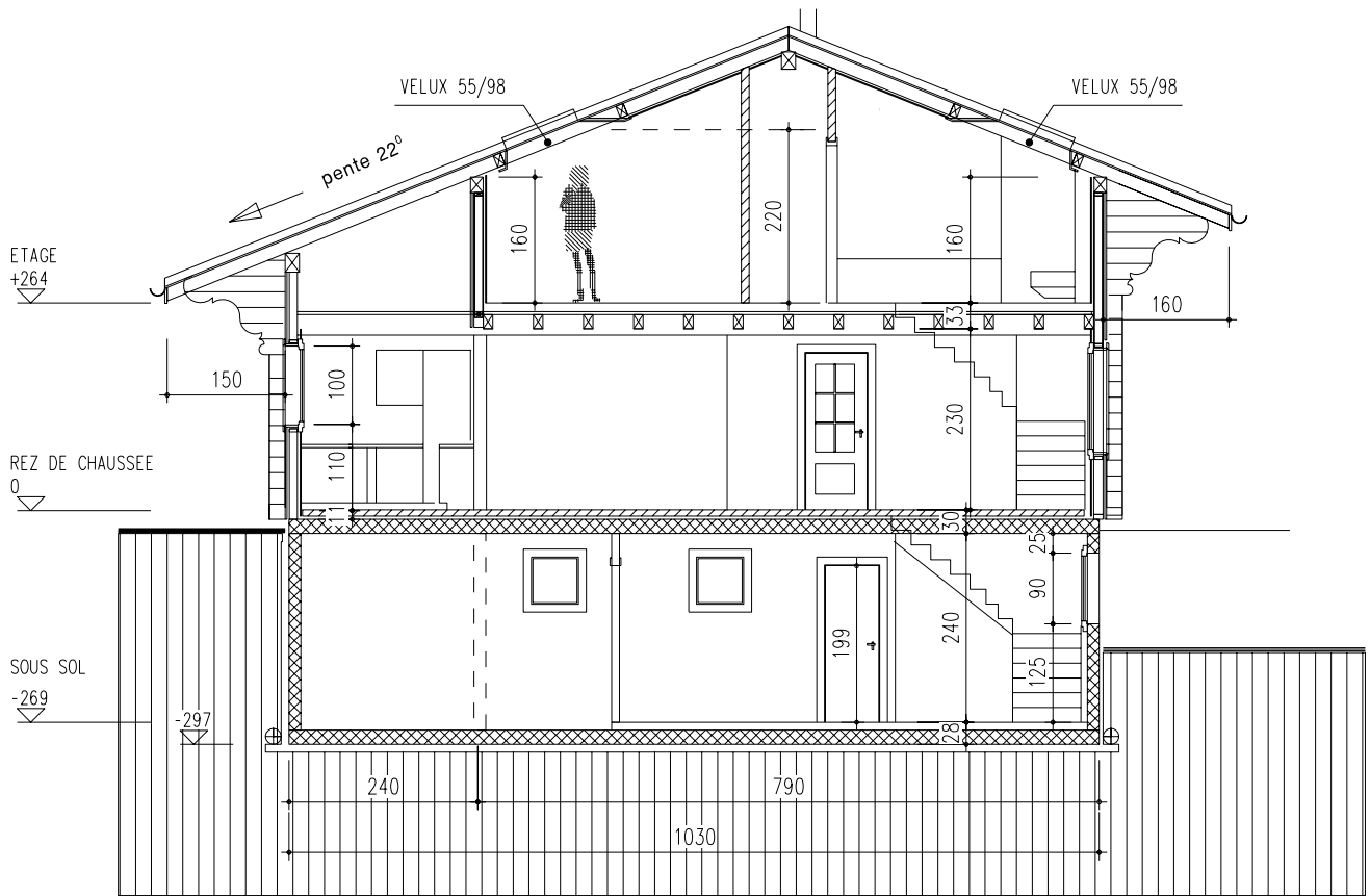
Coupe A-A
