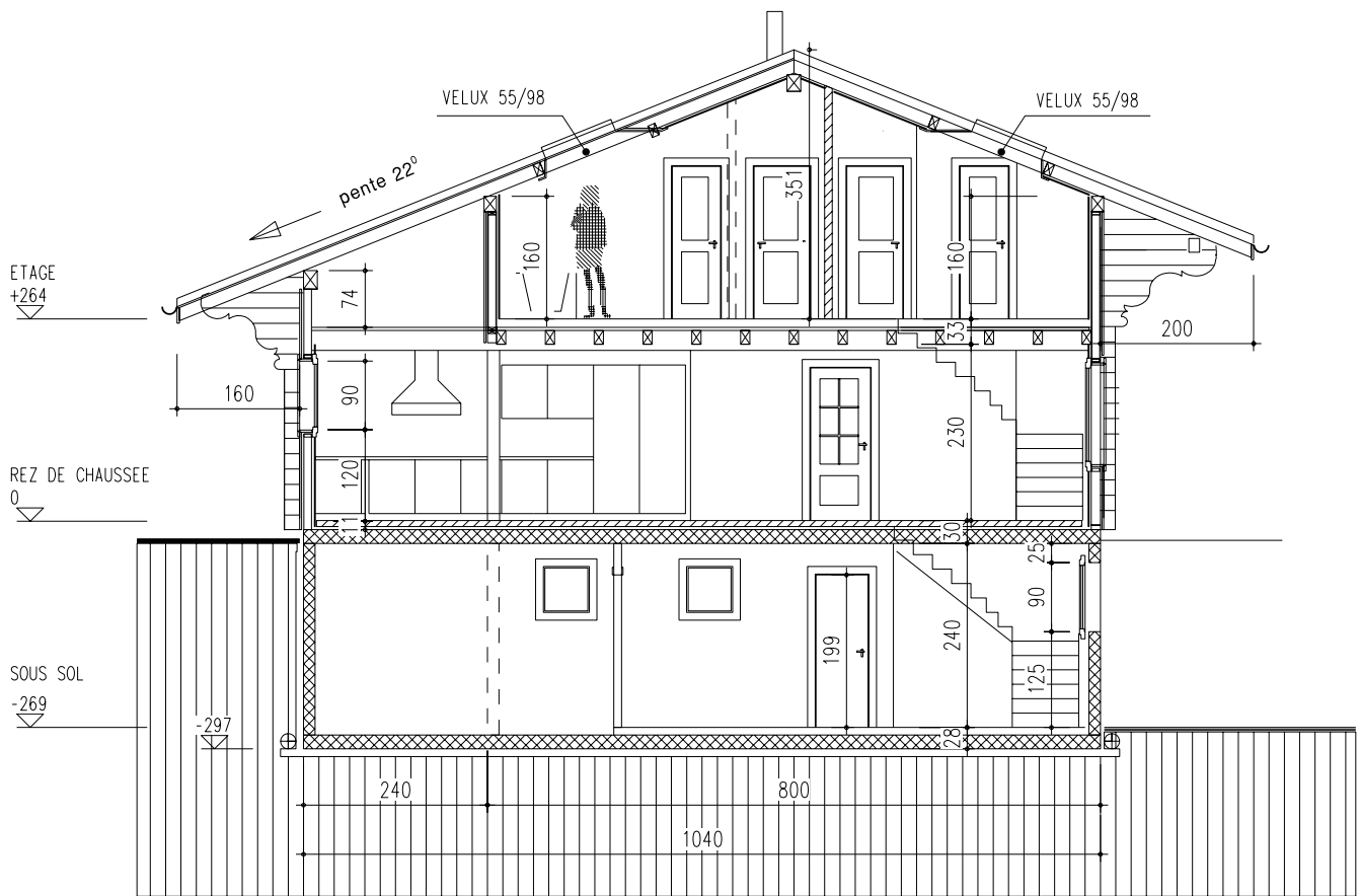
Coupe A-A
