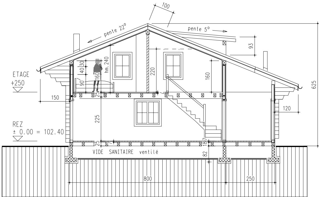
Coupe A-A
