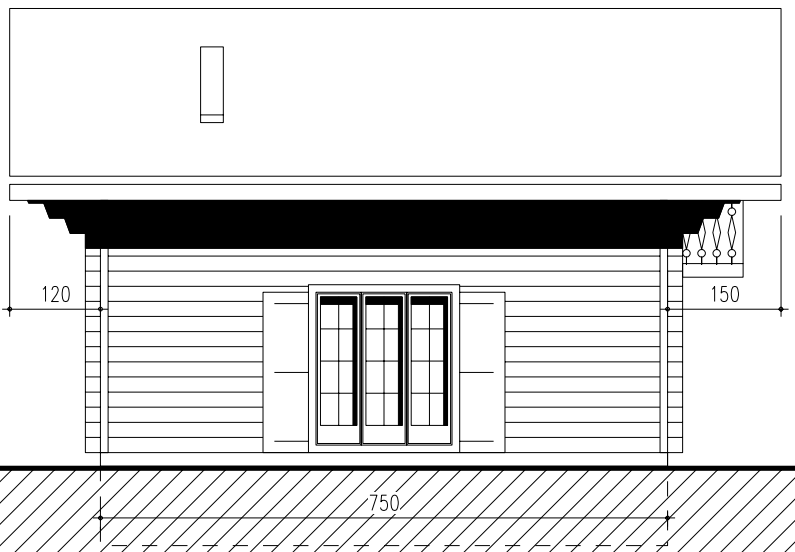
Facade Ouest
