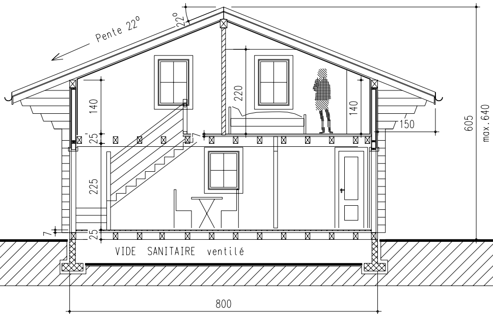
Coupe A-A
