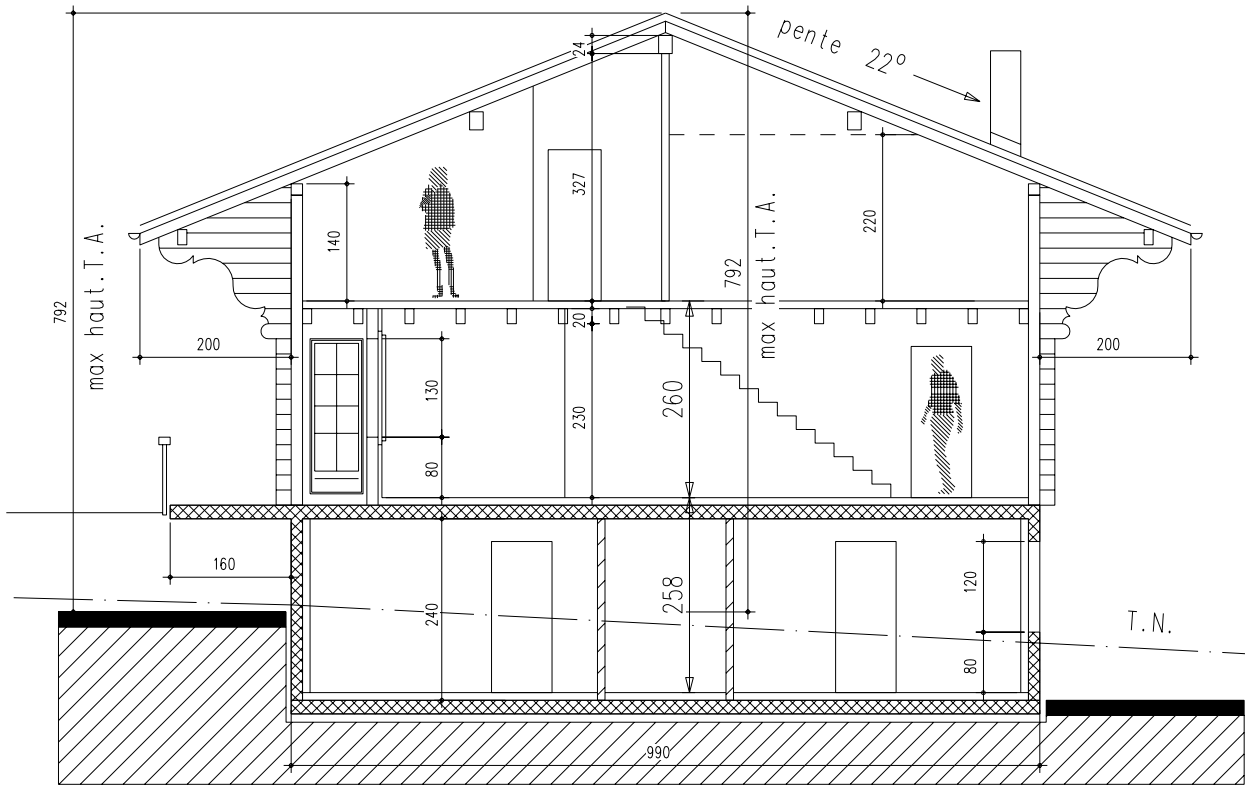
Coupe A-A
